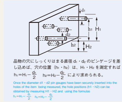
～穴の位置測定～ Hole Position Measurement
