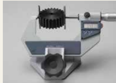
～歯車のオーバピン径測定～ Overpin diameter of gear
