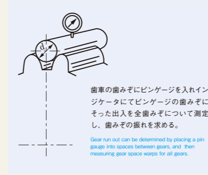
～歯車の歯みぞの振れの測定～ Gear Space Run Out Measurement
