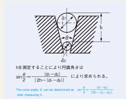
～傾斜角の測定(2)～ Angle of Inclination Measurement (2)
