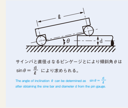
～傾斜角の測定(1)～ Angle of Inclination Measurement (1)
